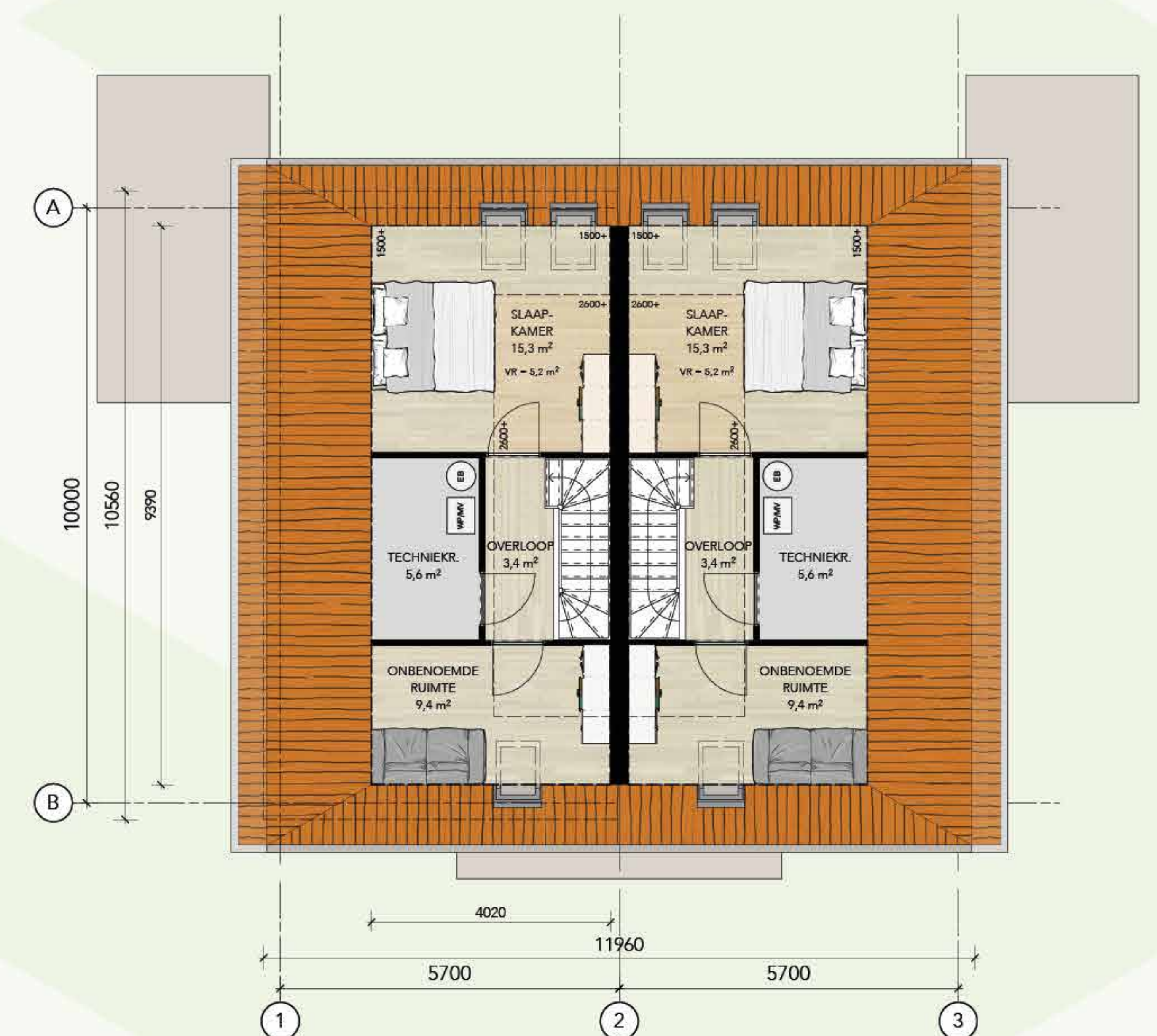
Tweede verdieping
