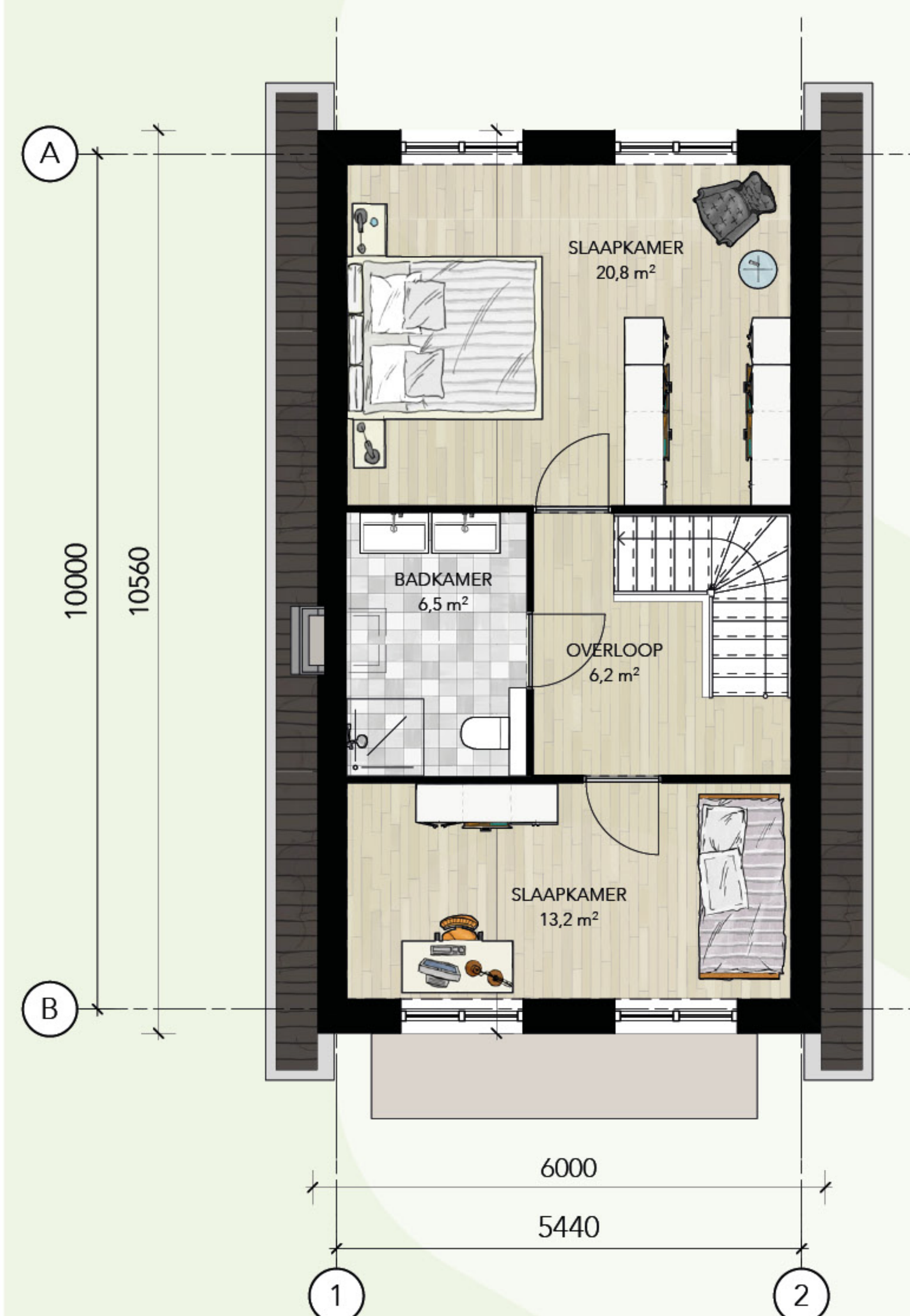
Eerste verdieping
