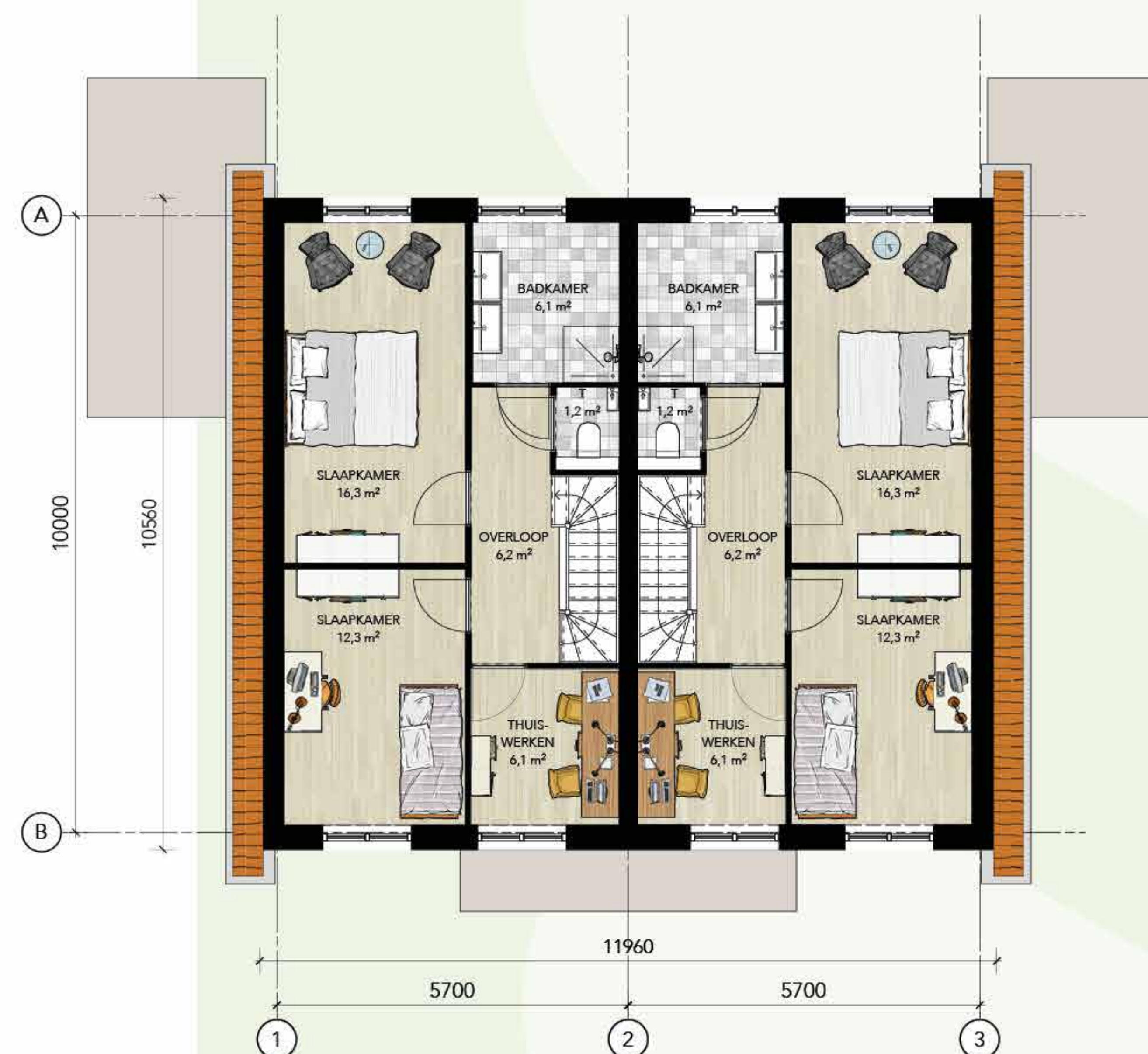
Eerste verdieping
