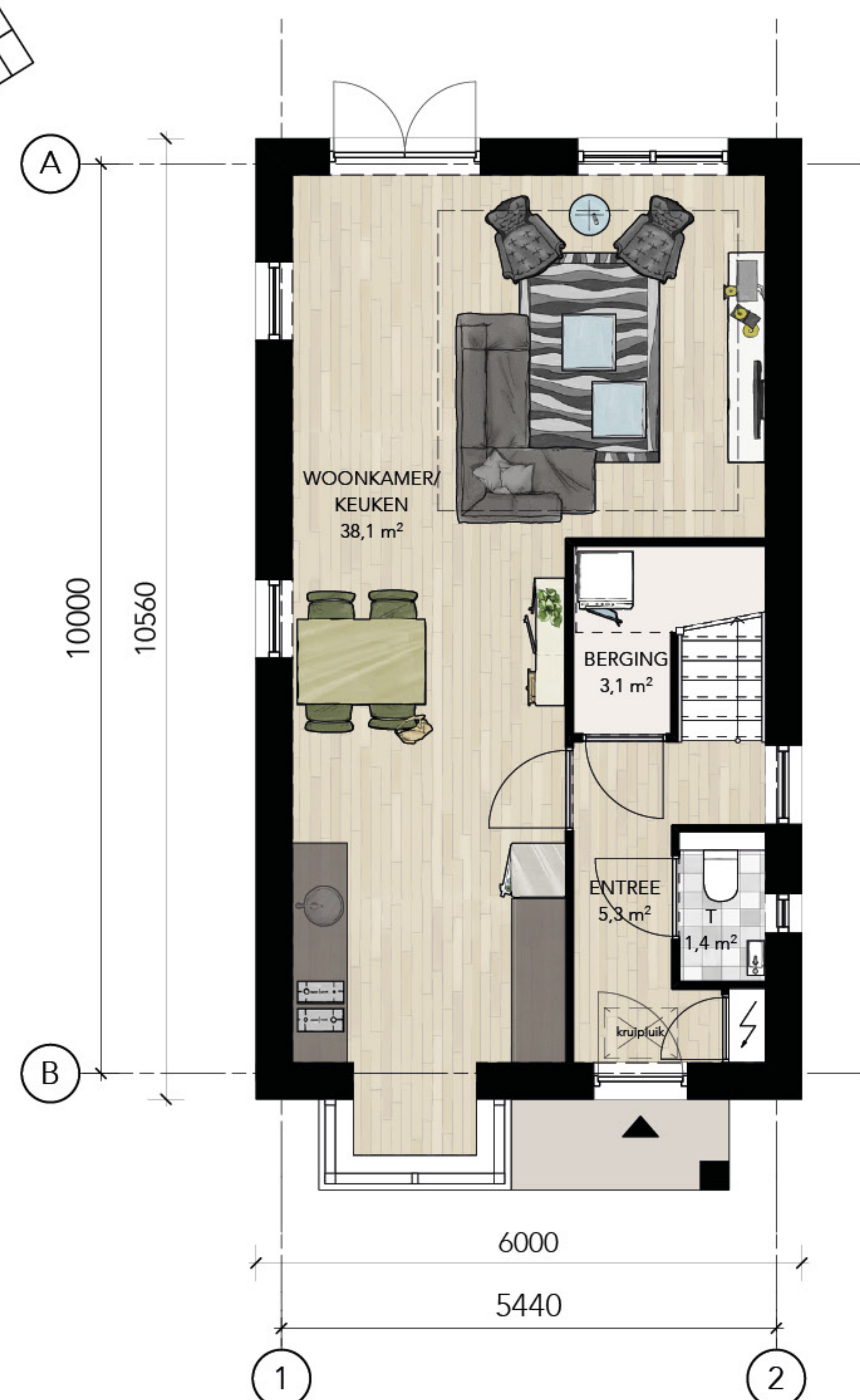
Begane grond
