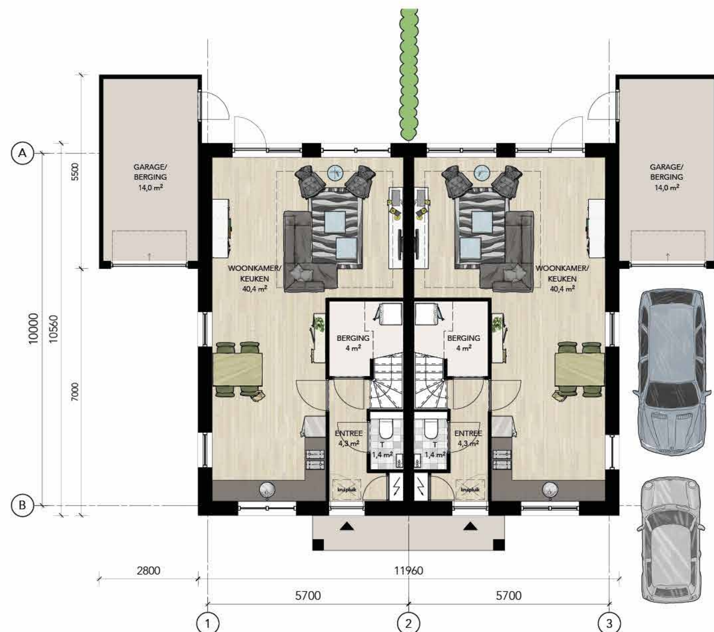
Begane grond
